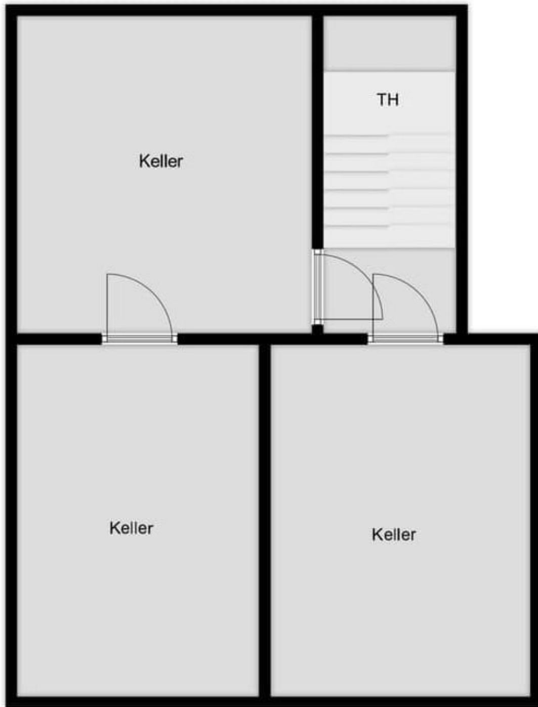
Kellergeschoss
